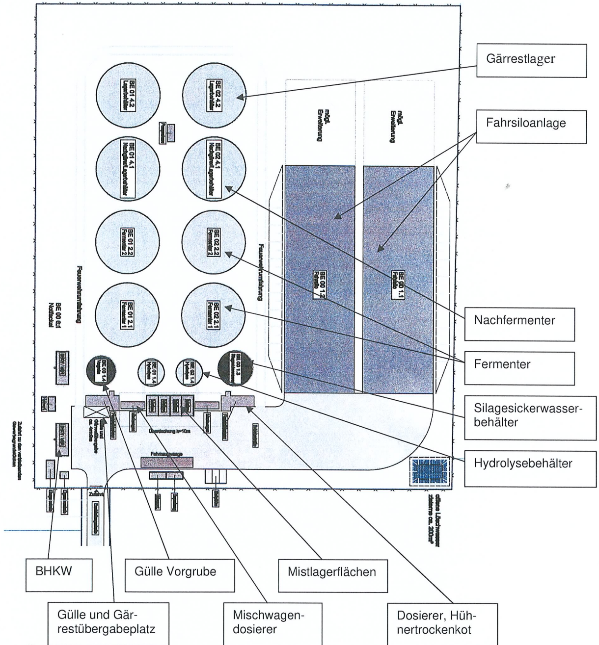
Bild 1: Aufbau der Biogasanlage
